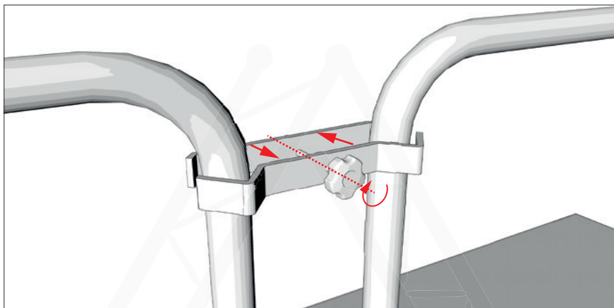
SCD-18 Klamra spinająca barierki handrails clamp
